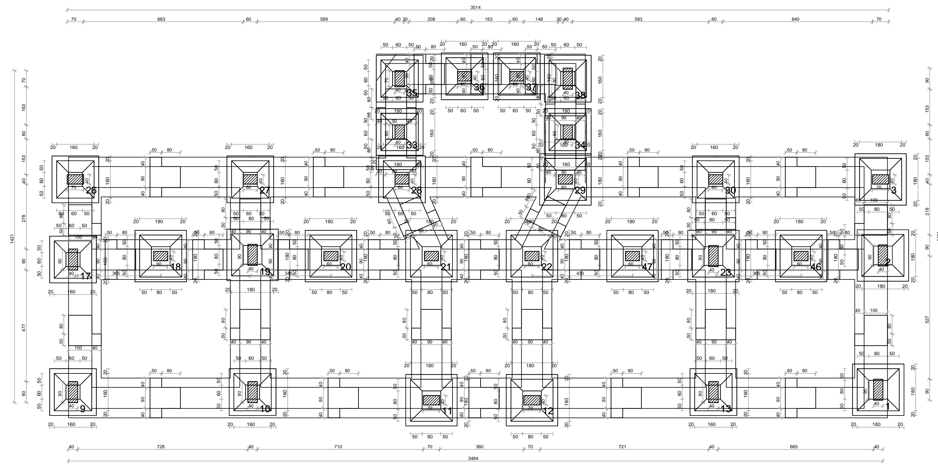
PIANTA IMPALCATO QUOTA m: 0.00
